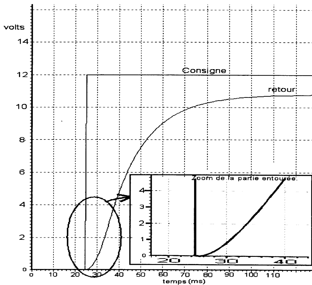
Graphe 1: Réponse en boucle ouverte.
